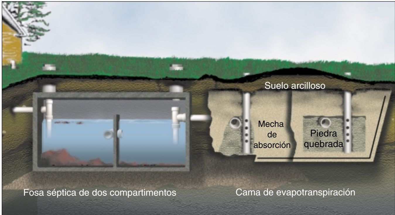
Figure 1: Un sistema de lecho de evapotranspiración.
