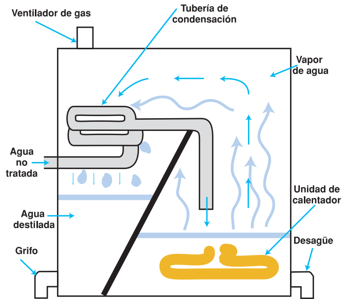
Figura 6. Proceso de destilación (adaptado de Kocher, et. al., 2003).
