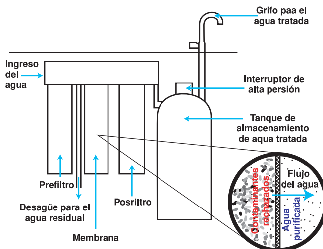
Figura 4. Unidad de tratamiento de osmosis inversa (adaptado de Kneen et al., 1995 y USEPA, 2003)
