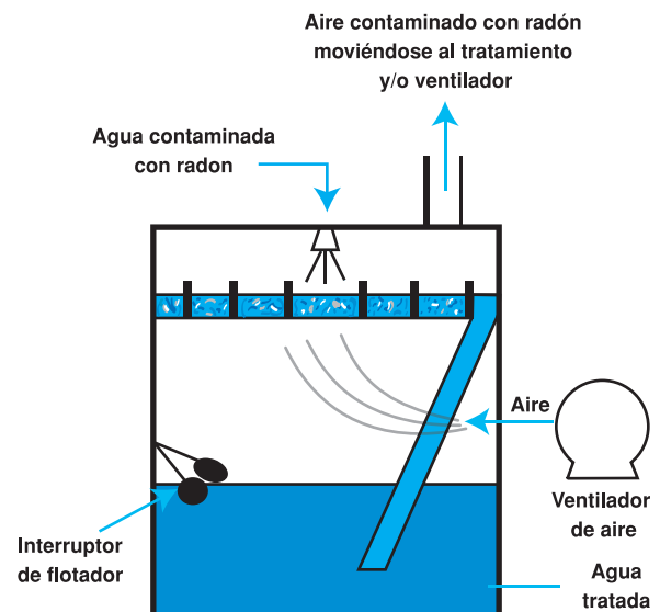
Figura 9. Sistema de aeración de bandeja superficial (adaptado de Twitchell, 2000).
