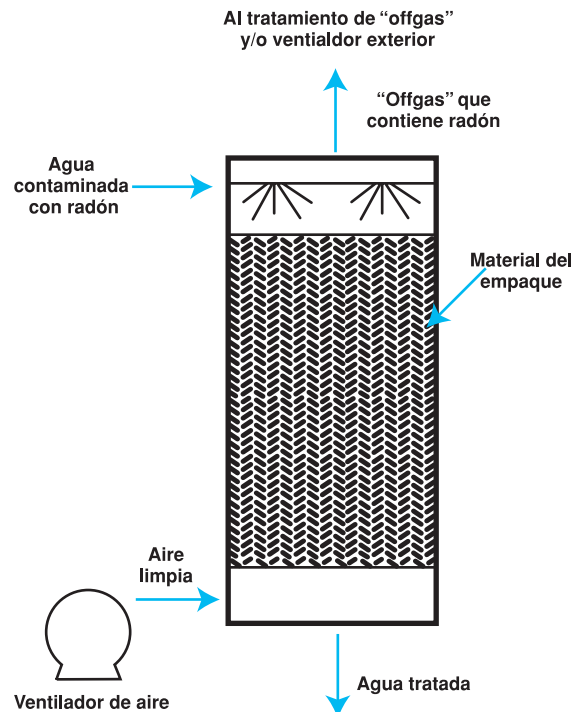
Figura 8. Sistema de aeración por columna empacada (adaptado de Robillard 2001a).
