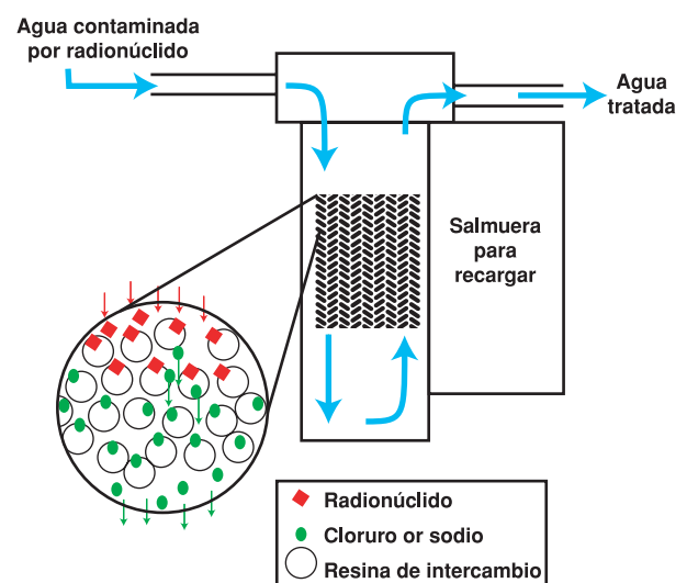
Figura 5. Proceso de intercambio de iones (adaptado de Robillard et al., 2001b).
