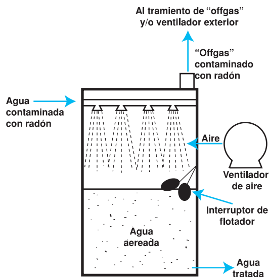
Figura 7. Sistema de aeración por rociado (adaptado de Robillard, 2001a).
