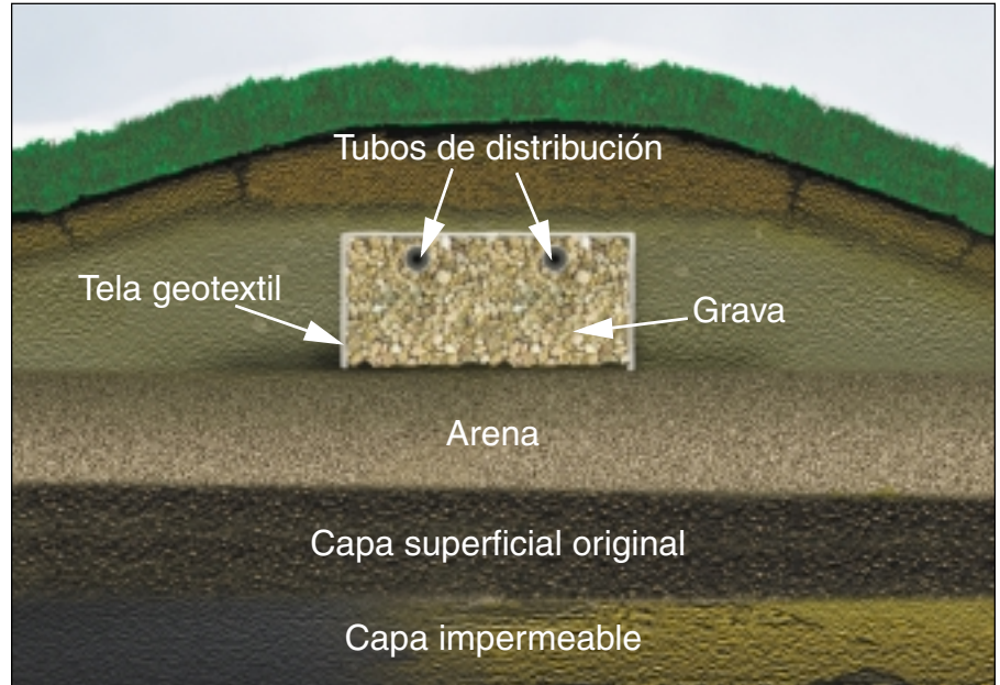
Figure 2: Un sistema de montículo se construye encima de la superficie natural del suelo.
