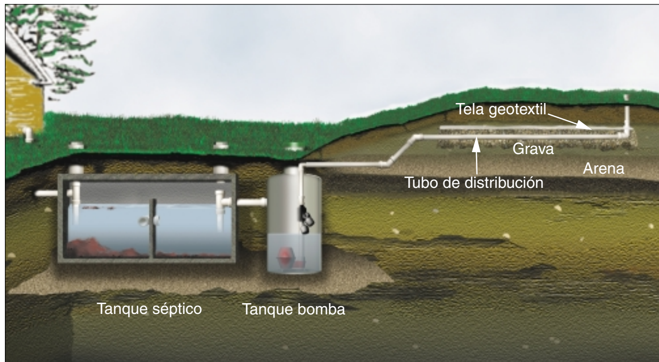
Figure 1: Un sistema de montículo para distribuir aguas negras tratadas al suelo.
