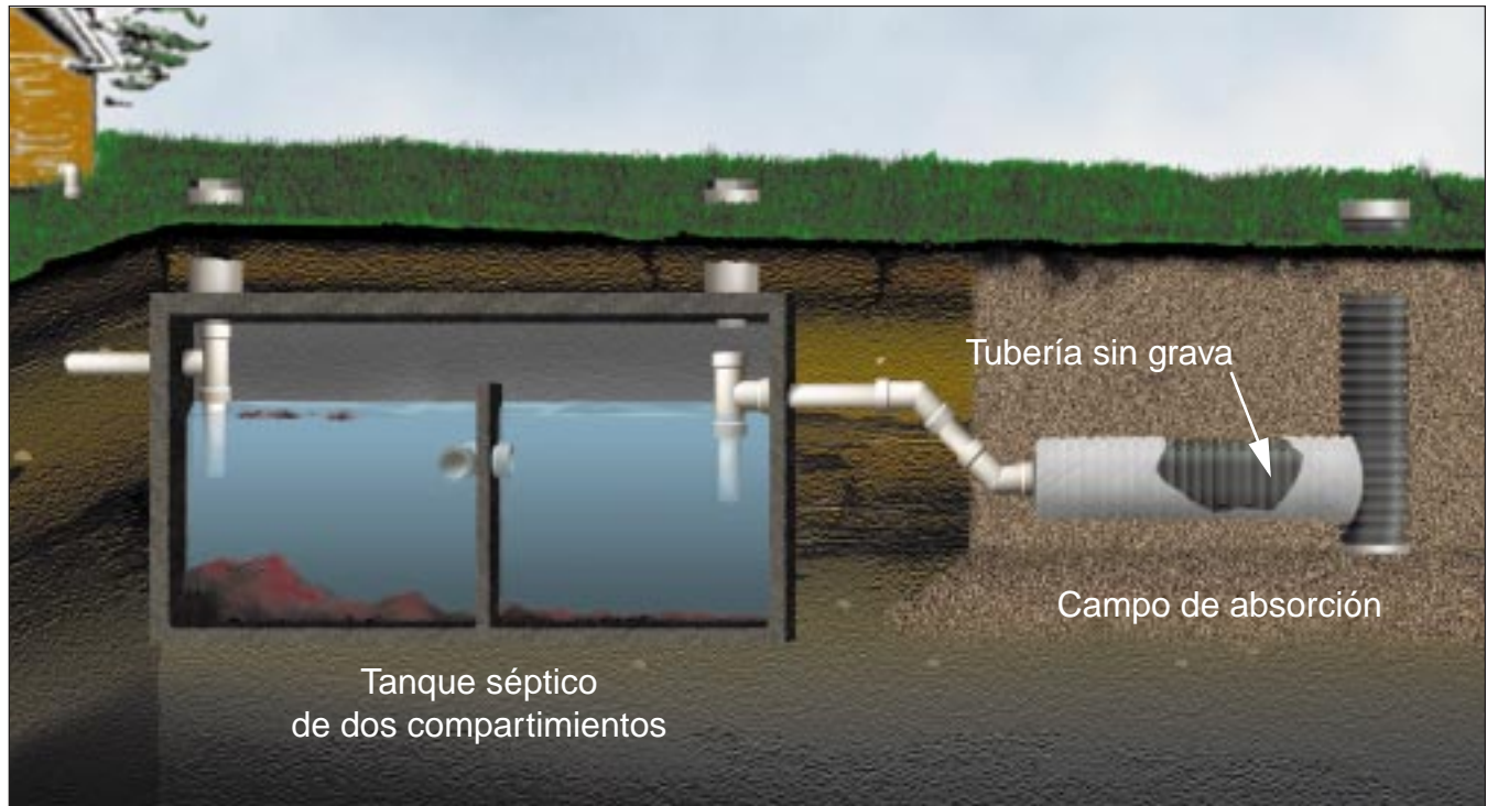
Figura 1: La tubería sin grava es flexible y puede ponerse en zanjas siguiendo las curvas a nivel en suelos con pendiente.
