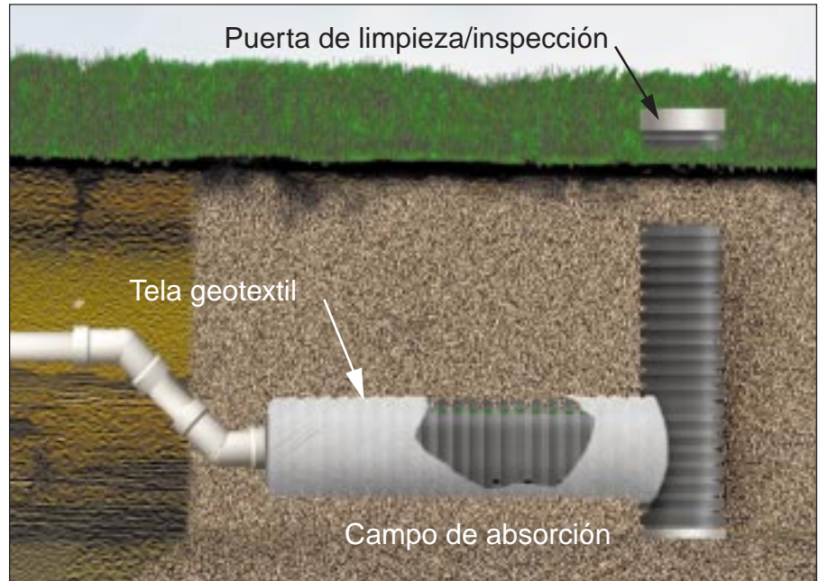
Figura 2: La tubería sin grava está rodeada de tela geotextil en lugar de grava.
