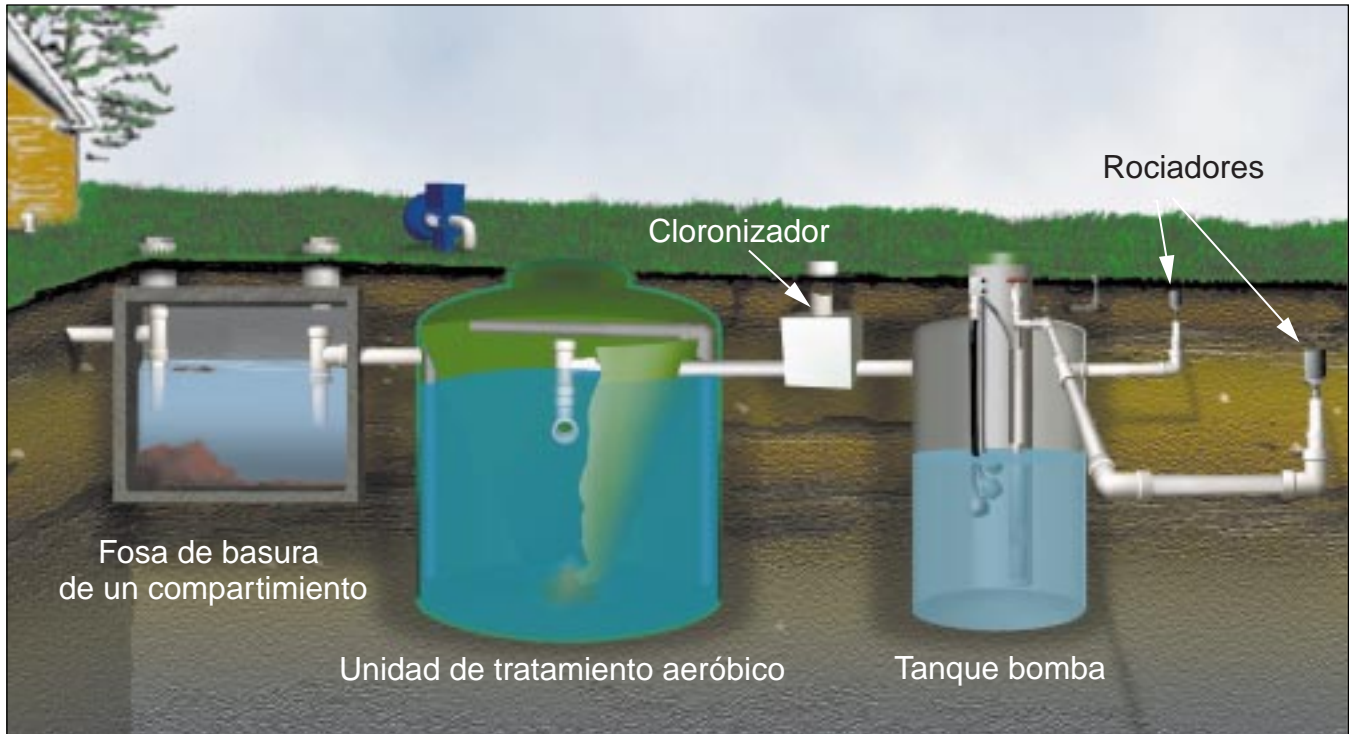
Figura 1: Un sistema individual para el tratamiento de agua negra con una unidad de tratamiento aeróbico.
