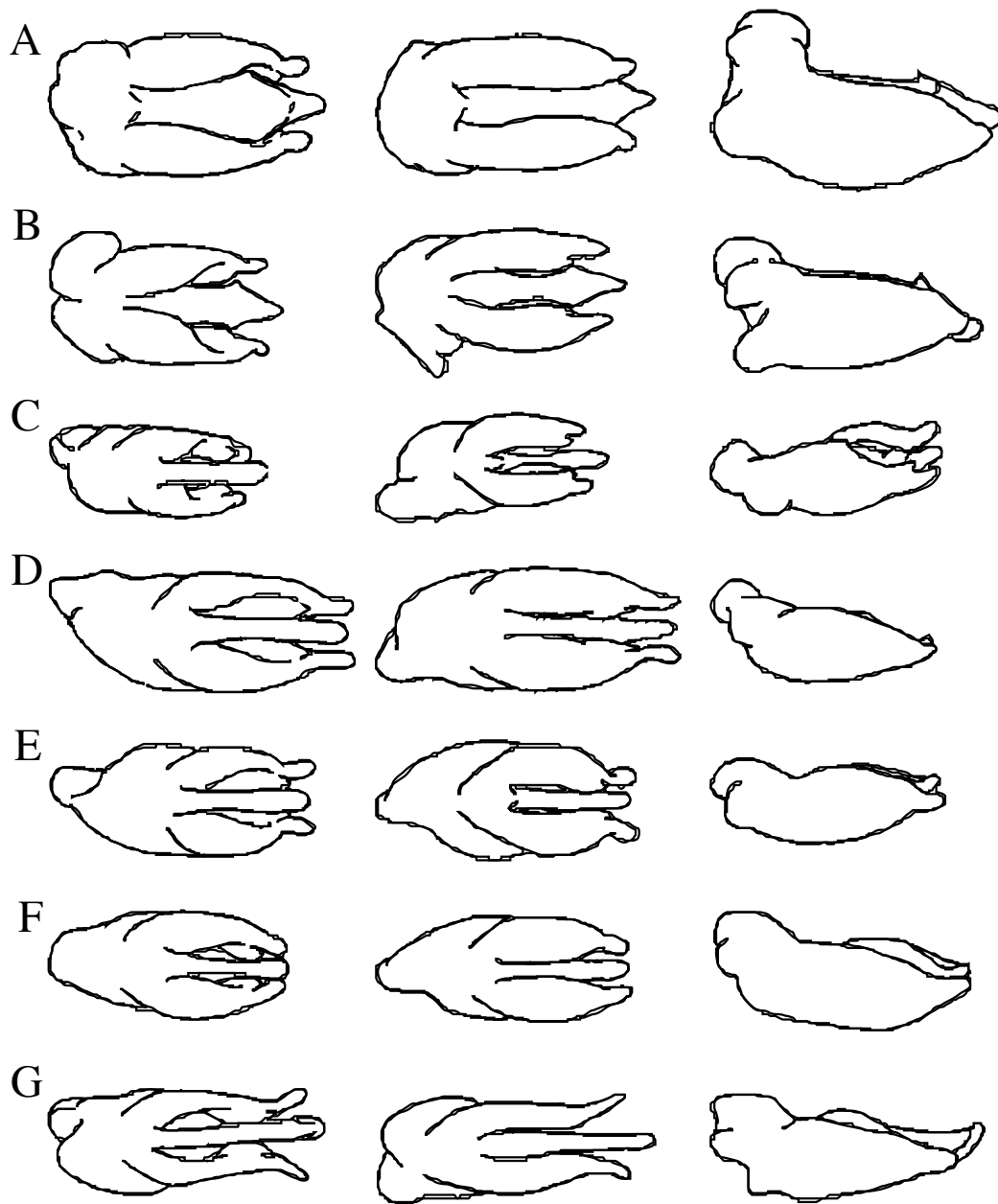
Fig 2. Genitalia of Microphotus . Dorsal, ventral and lateral view from left to right. A= M. chiricahuae , B= M. pecosensis , C= M. octarthrus , D= M. dilatatus , E= M. deacrthus , F= M. fragilis , G= M. angustus
