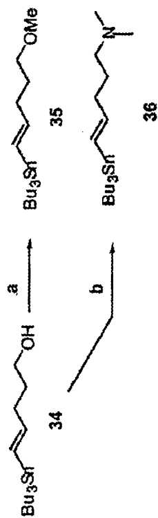
Scheme 3. a. \text{Ag}_2\text{O} , MeI, \text{CH}_3\text{CN} , reflux, 9 h, 25%; b. i) TsCl, py., \text{CH}_2\text{Cl}_2 , 0 °C, 8 h, 65% ii) dimethyl amine (E), THF, -78 °C, 6 h, 85%.
