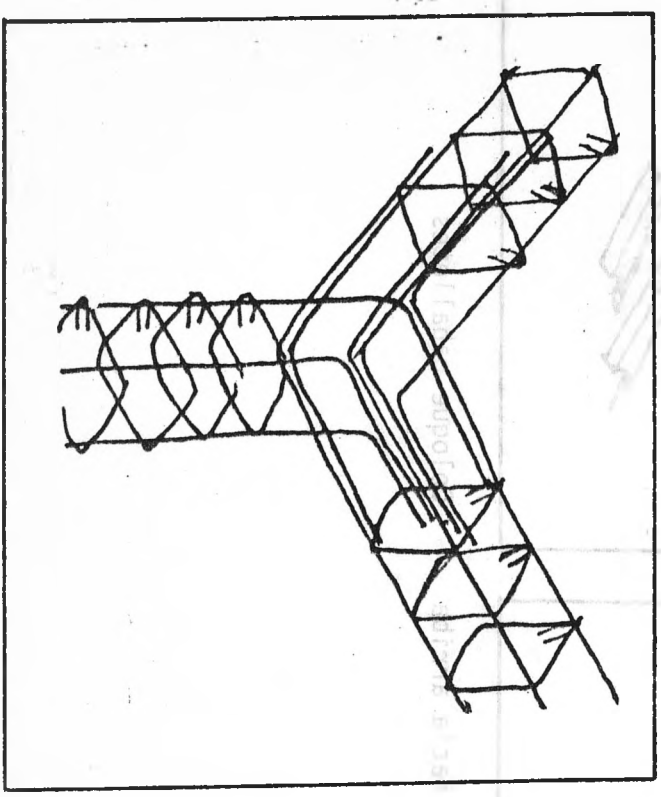
Unión de columneta con vigas de amarre en esquina
